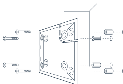
РИС. 2. Схема монтажа крепежной панели SmartBracket
