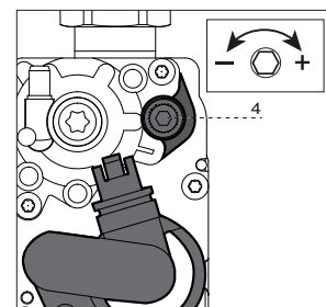
Газовий клапан 8205
