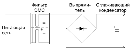
Рис. 57 Выпрямление напряжения переменного тока в напряжение постоянного тока
