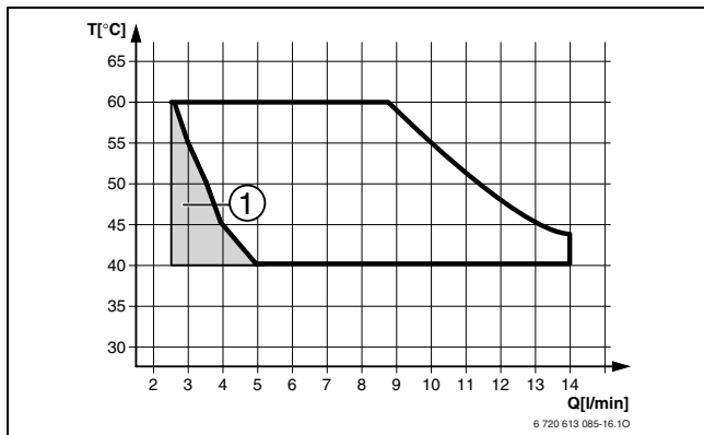
Рис. 11 Діаграма для холодної води на вході від +15 °C (ZWC 28-3 MFA/MFK)
