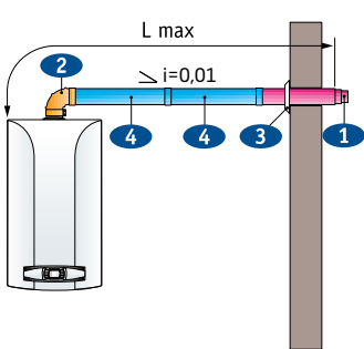
Коаксіальний димар з горизонтальним виводом через стіну
