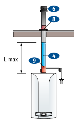
Коаксіальний димар з вертикальним виведенням на плоский дах
