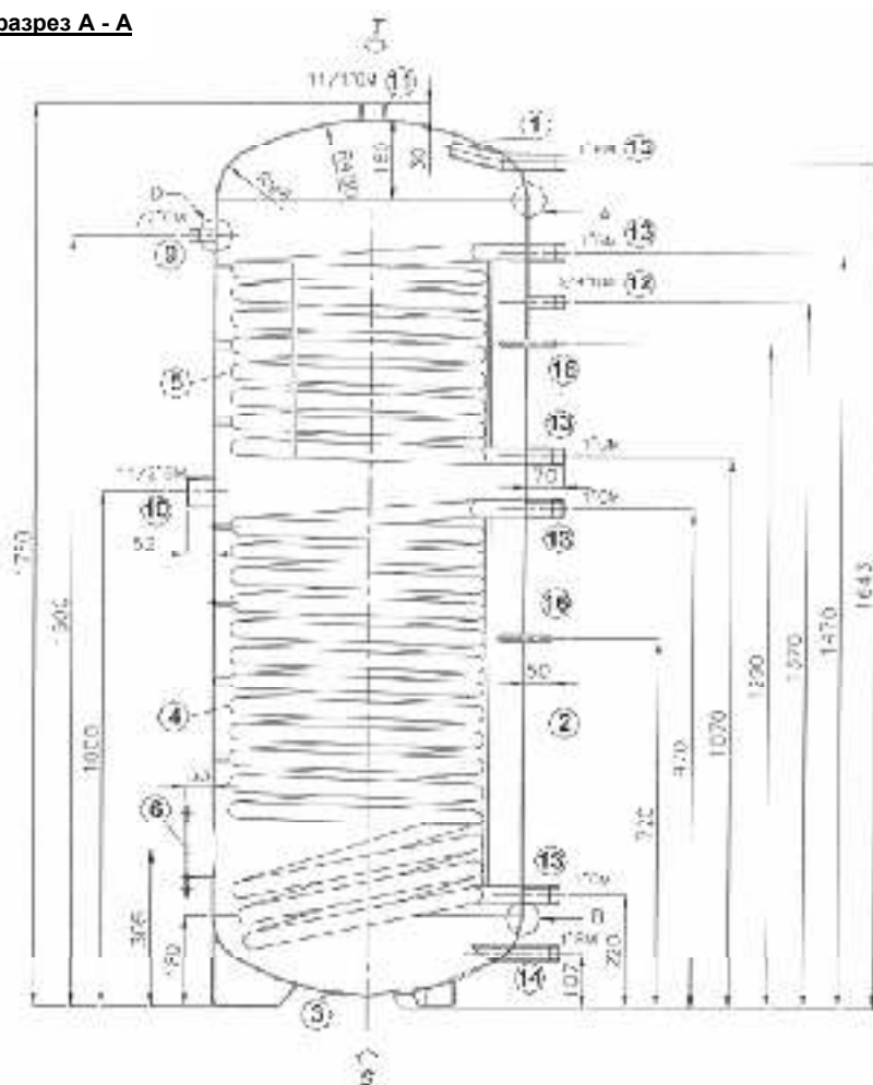
ФРОНТАЛЬНЫЙ РАЗРЕЗ
