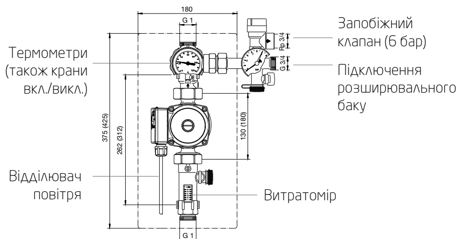
Сонячна гідростанція з однією лінією (насосною)
