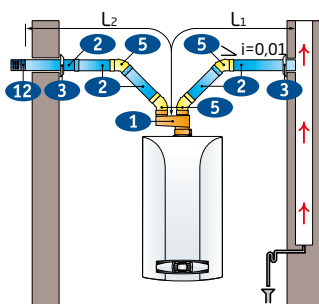
Роздільні труби з виведенням димової труби в димар і забором повітря з вулиці
