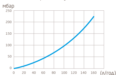
Втрати тиску SB20+V
