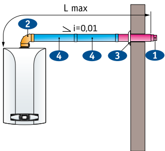
Коаксіальний димар з горизонтальним виводом через стіну
