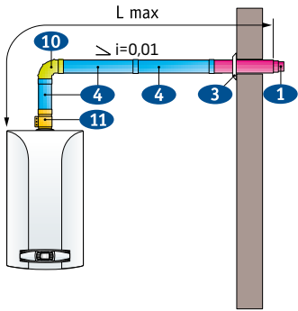
Коаксіальний димар з горизонтальним виводом через стіну
