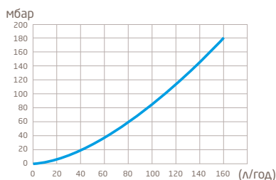
Втрати тиску SB20+O
