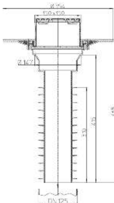
Рис. 3. Кровельная воронка HL69BP/2.
