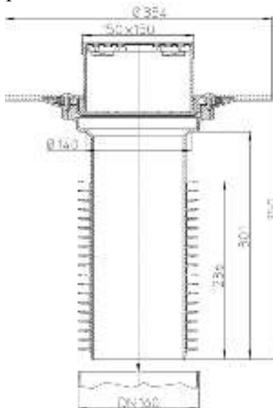
Рис. 3. Кровельная воронка HL69BP/2.
