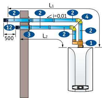
Роздільні труби з приєднанням до єдиної системи димовиведення і повітрязабору
