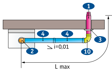
Коаксіальний димар з горизонтальним виводом через стіну
