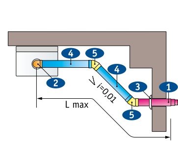
Коаксіальний димар з горизонтальним виводом через стіну
