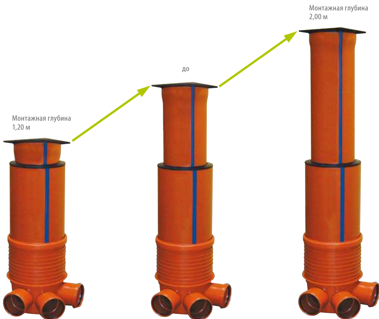
Система колодцев – компакт DN 400 с телескопической трубой и крышкой
