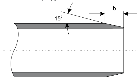
Рис. 3а Скол на конце трубы
