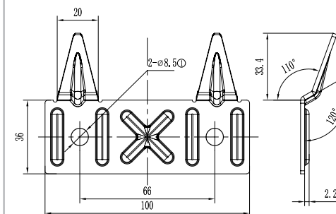
Монтажная планка размеры, мм
