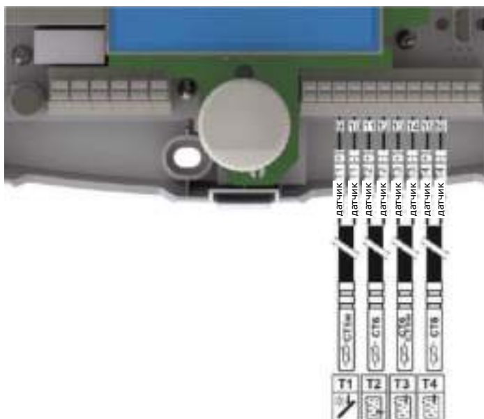
Рис. 16-8 Подключение датчиков температуры*
