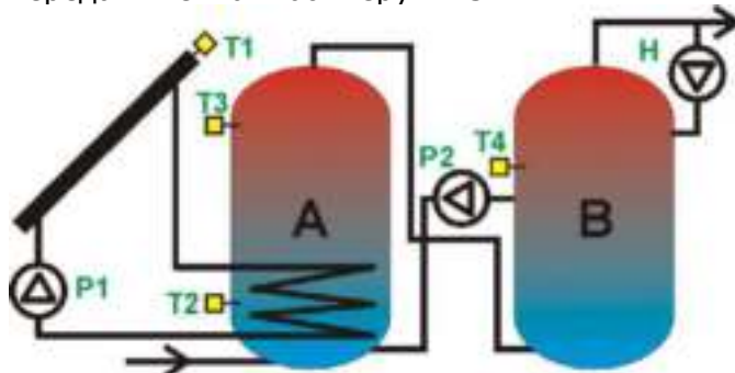
Рис. 13-4 Гидравлическая схема D
