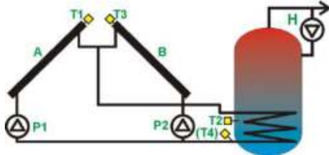
Рис. 13-8 Гидравлическая схема Н
