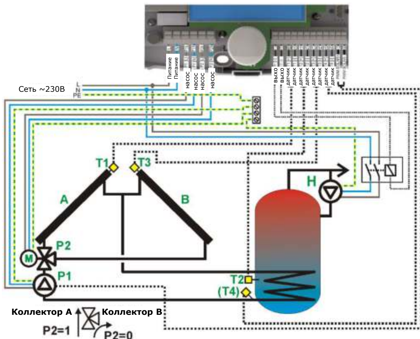
Рис. 17-12 Гидравлическая схема L
