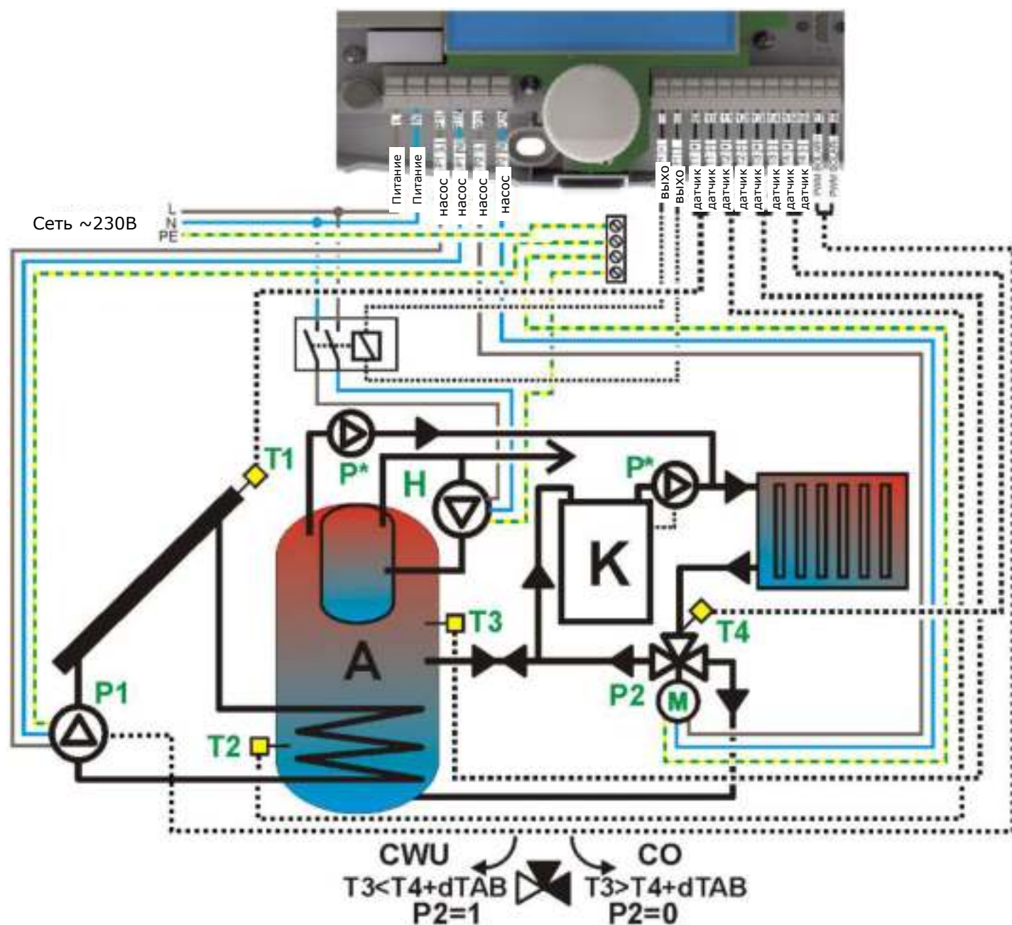
Рис. 17-11 Гидравлическая схема К
