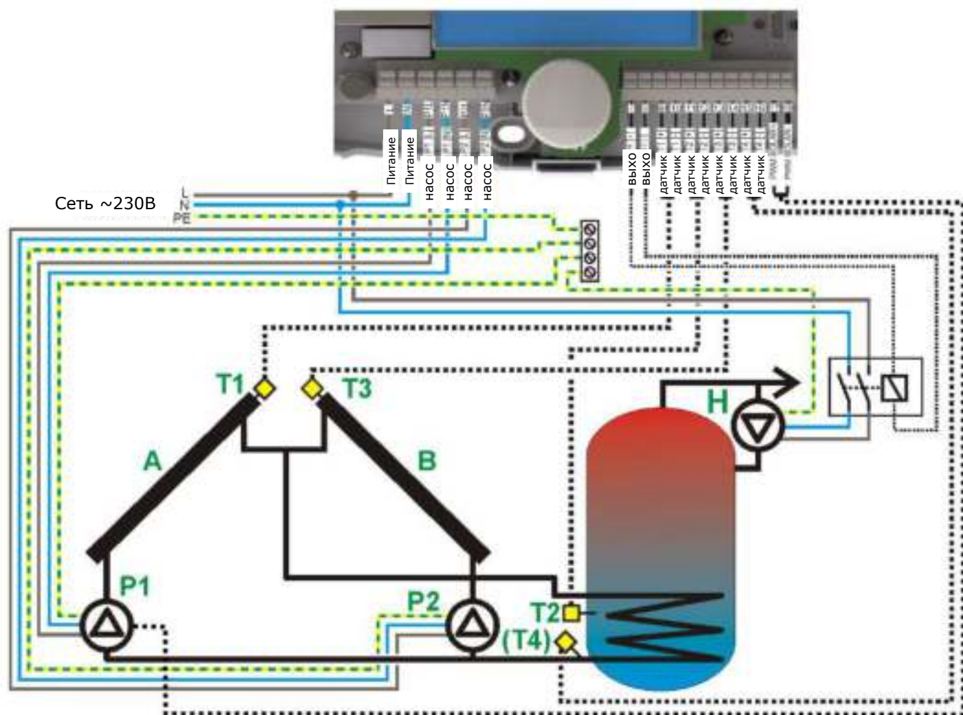
Рис. 17-8 Гидравлическая схема Н
