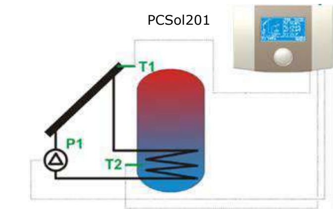
Рис. 2-1 Базовая гидравлическая схема
