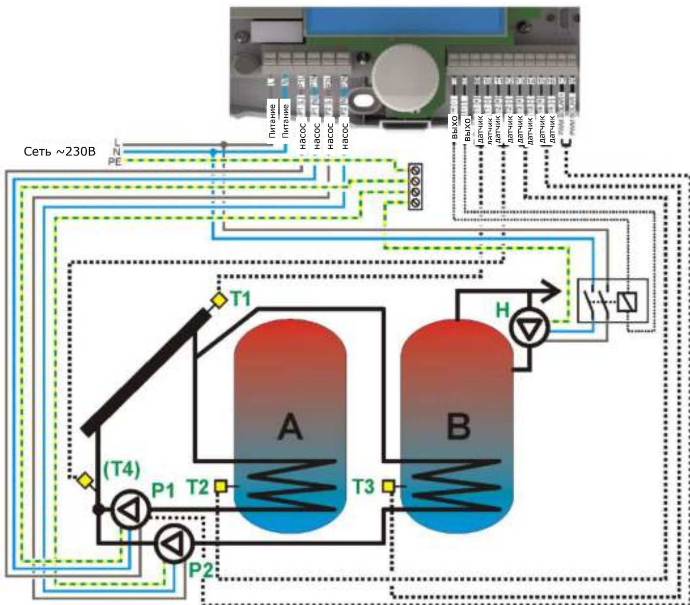
Рис. 17-5 Гидравлическая схема Е
