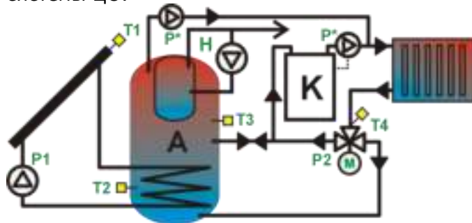
Рис. 13-11 Гидравлическая схема K
