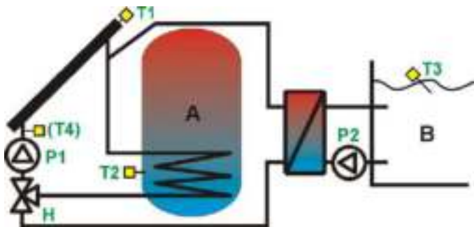
Рис. 13-6 Гидравлическая схема F
