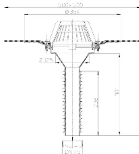
Рис. 1. Кровельная воронка HL69H/7.
