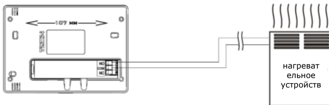
1 Схема подключения регулятора ST-290 непосредственно с нагревательным устройством.
