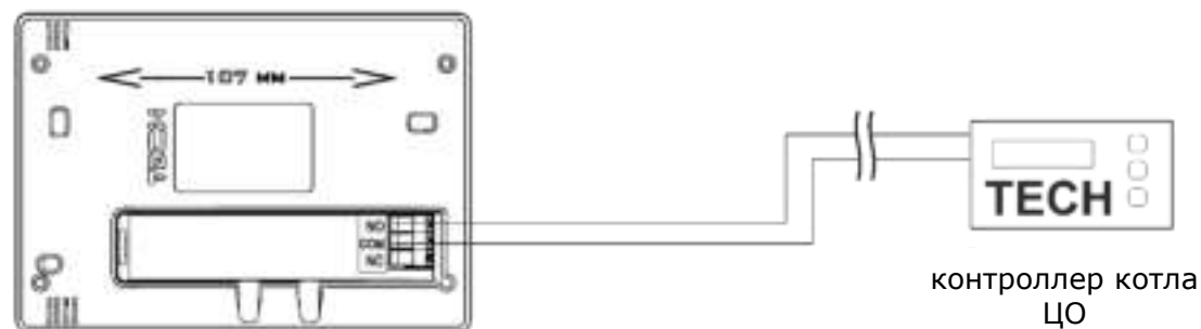
1 Схема подключения регулятора ST-290 непосредственно с нагревательным устройством.
