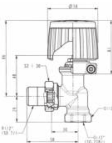
FJVR 15 (1/2"), кутовий клапан
