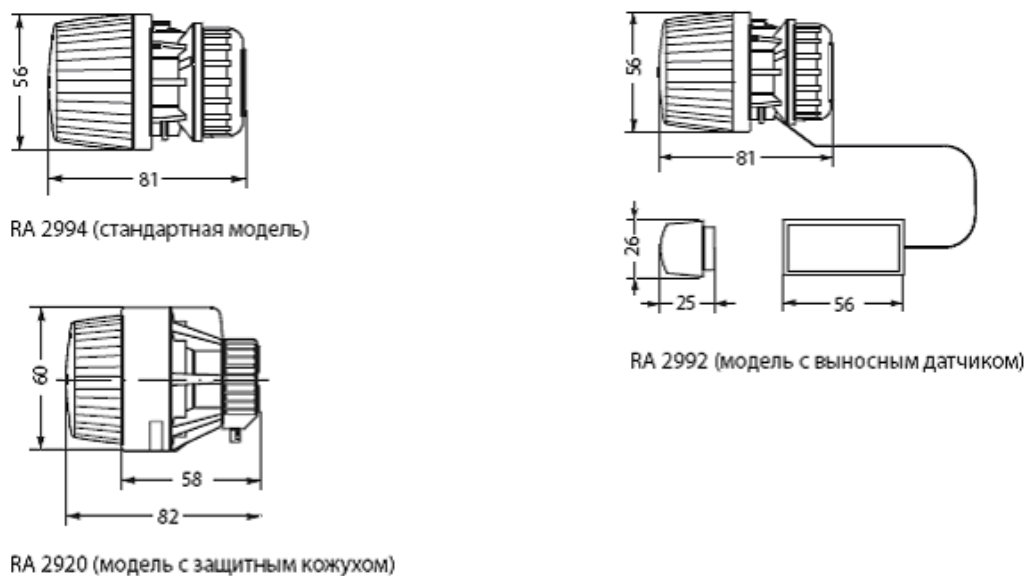
Рис. 2. Габаритные размеры термозадающих элементов модификаций RA 2920, 2992, 2994
