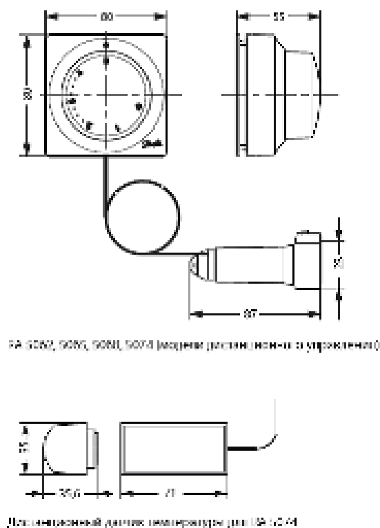
Рис.3. Габаритные размеры термозадающих элементов модификаций RA 5062, 5065, 5068, 5074 и датчика температуры
