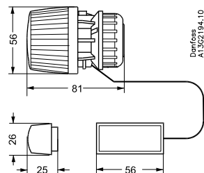
Модель з виносним датчиком RA 2992
