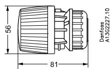
Стандартне виконання RA 2991
