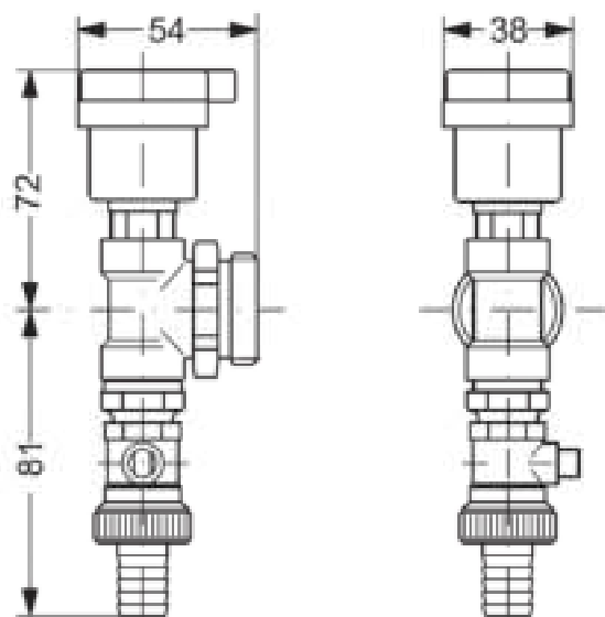
Рис. 6. Воздушный клапан автоматический типа FHF-EA.
