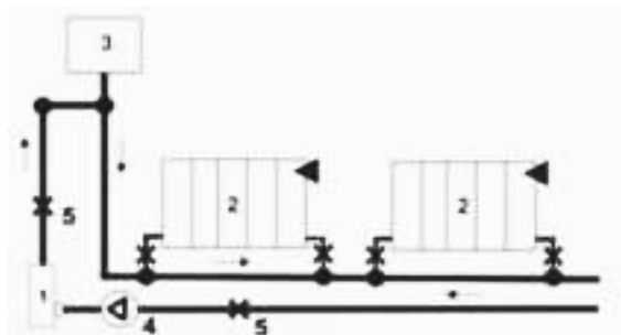
Рис. 1 –Схема однопроходной системы водяного отопления с принудительной циркуляцией
