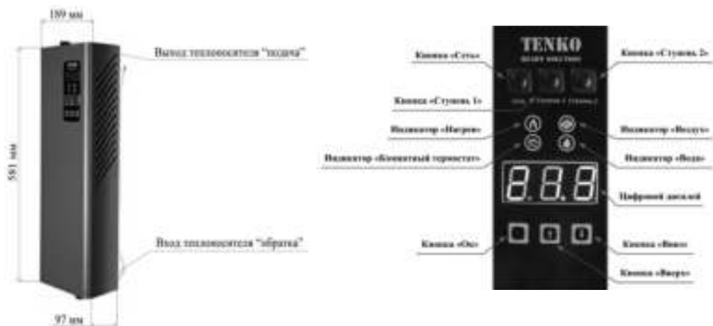
Рис.2. Внешний вид электродотла Tenko «Standart Digital»
