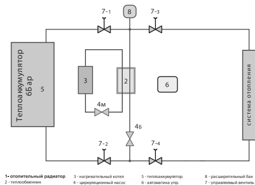
Рис.10. Схема с использованием теплоаккумулятора рассчитанным под высокие давления (6÷10 Бар). Давление в теплоаккумуляторе соответствует давлению в системе.
