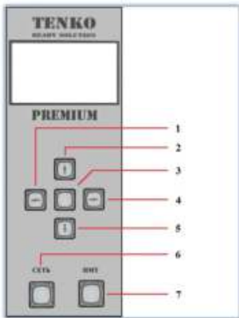
Рис. 5 – Лицевая панель котла
