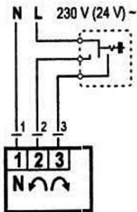
Трьохконтактний термостат
