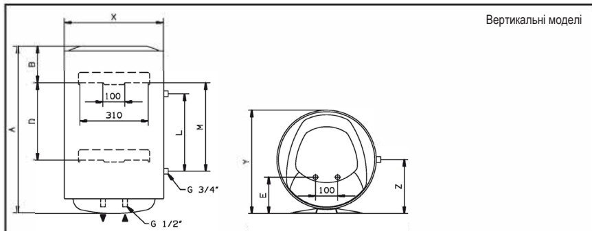
Схема установки
