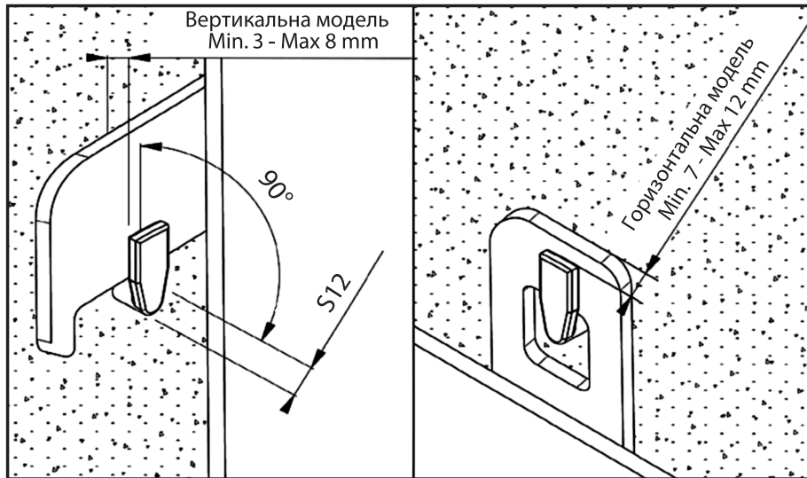
Схема установки
