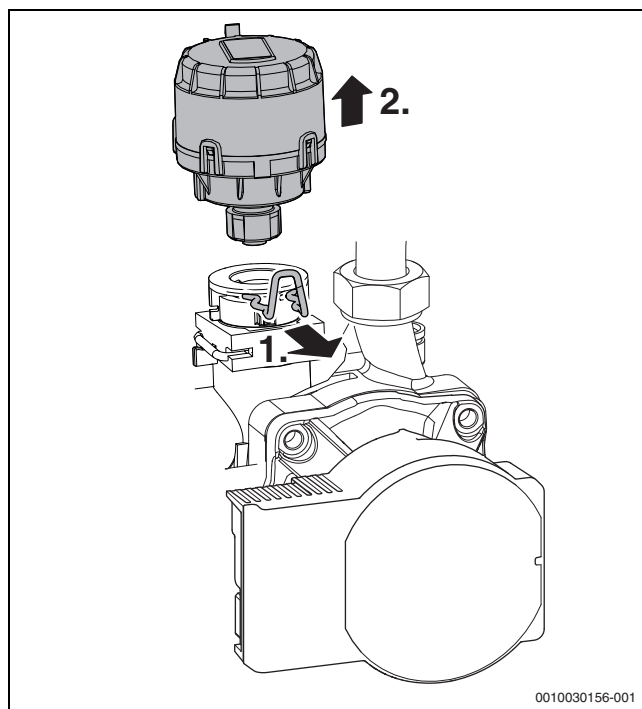
Рис. 103 Демонтаж двигателя 3-ходового клапана
