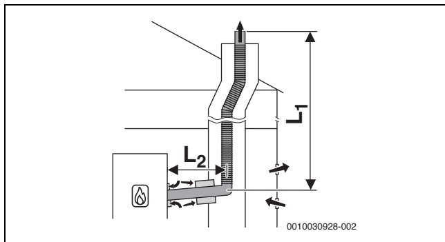
Рис. 47 Схема гибкого отвода дымовых газов в шахте согласно B 53p с забором воздуха из помещения топочной для подвода воздуха и с концентрическим соединительным элементом между помещением для установки и шахтой
