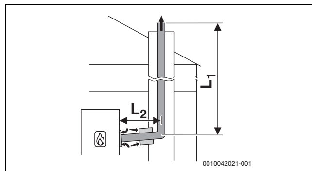
Рис. 40 Жёсткий отвод дымовых газов в шахте по B 53p с забором воздуха из помещения и с концентрическим соединительным элементом между помещением установки котла и шахтой
