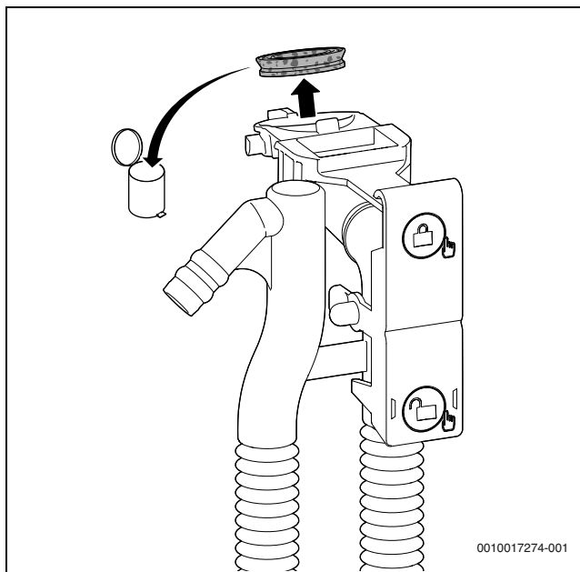
Рис. 92 Демонтаж уплотнения сверху на сифоне для отвода конденсата
