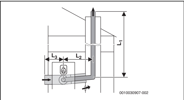
Рис. 23 Схема жесткого отвода дымовых газов согласно C 53x в шахте и схема подачи воздуха/отвода дымовых газов с отдельной линией подвода воздуха и концентрической линией отвода дымовых газов в помещении для установки
