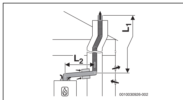
Рис. 41 Схема гибкого отвода дымовых газов в шахте согласно B 53p с забором воздуха из помещения топочной для подвода
