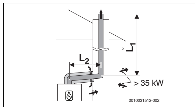
Рис. 48 Схема жесткого отвода дымовых газов в шахте согласно B 33 с забором воздуха из помещения через концентрический подвод воздуха/отвод дымовых газов в помещении для установки
