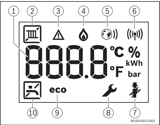
Рис. 71 Показания на дисплее
