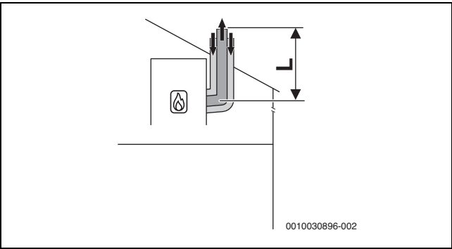
Рис. 15 Вертикальная концентрическая схема подачи воздуха/отвода дымовых газов согласно C 33x
