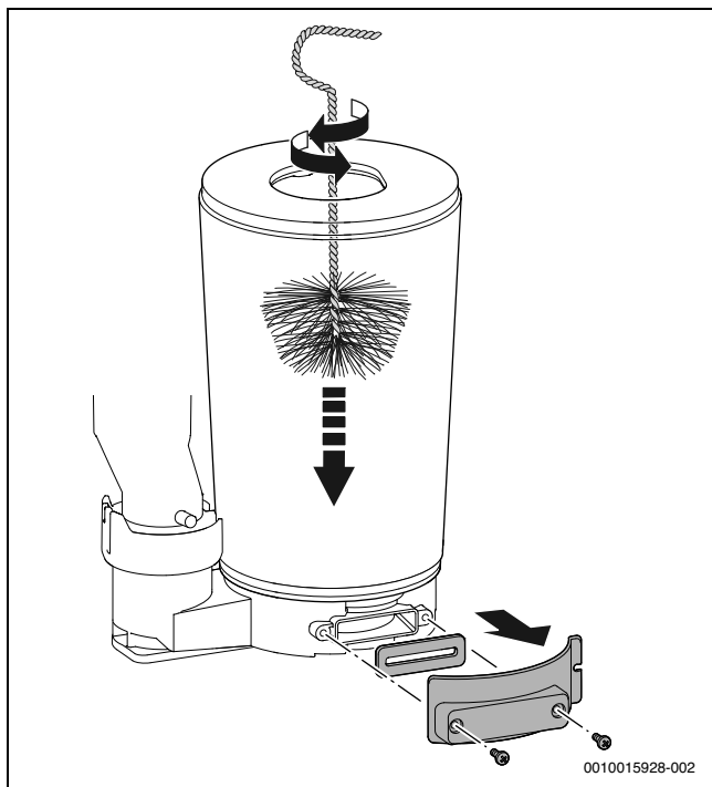
Рис. 87 Чистка теплообменника
