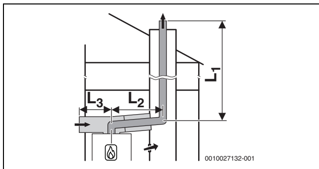
Рис. 26 Схема жесткого отвода дымовых газов согласно C 53x в шахте и схема подачи воздуха/отвода дымовых газов с отдельной линией подвода воздуха и concentricкой линией отвода дымовых газов в помещении для установки
