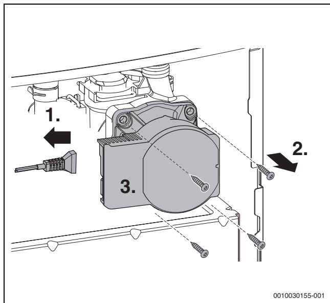
Рис. 101 Демонтаж насоса отопительного контура
