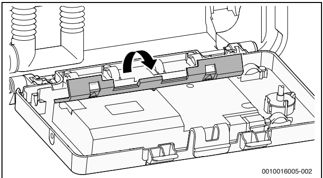
Рис. 68 Открывание пластиковой крышки
