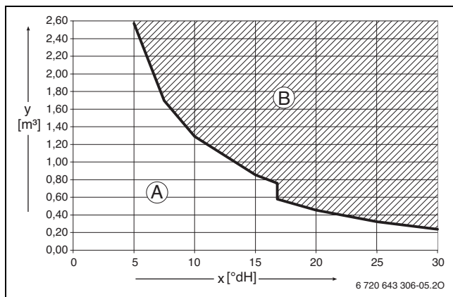
Рис. 59 Требования к воде для заполнения и подпитки в °dH для котлов < 50 кВт
