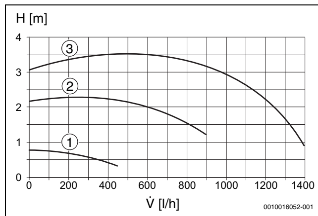
Рис. 75 Характеристическая кривая насоса отопительного контура (пропорциональное давление)
