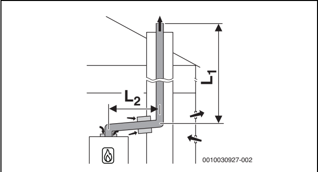
Рис. 44 Жёсткий отвод дымовых газов в шахте по B 53p с забором воздуха из помещения и с концентрическим соединительным элементом между помещением установки котла и шахтой
