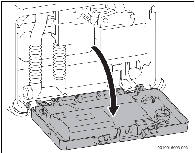
Рис. 67 Откидывание электронного блока вниз
