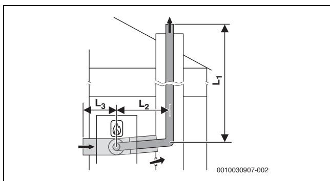
Рис. 27 Схема жесткого отвода дымовых газов согласно C 53x в шахте и схема подачи воздуха/отвода дымовых газов с отдельной линией подвода воздуха и concentricкой линией отвода дымовых газов в помещении для установки
