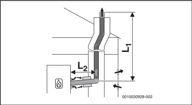
Рис. 42 Схема гибкого отвода дымовых газов в шахте согласно B 53p с забором воздуха из помещения топочной для подвода воздуха и с концентрическим соединительным элементом между помещением для установки и шахтой
