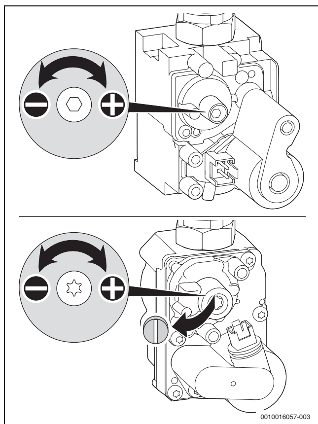
Рис. 77 Снятие пломбы с регулировочного винта
