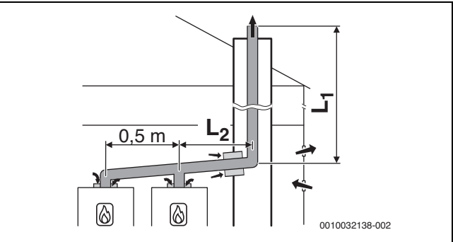
Рис. 56 Схема каскада с 2 котлами:
