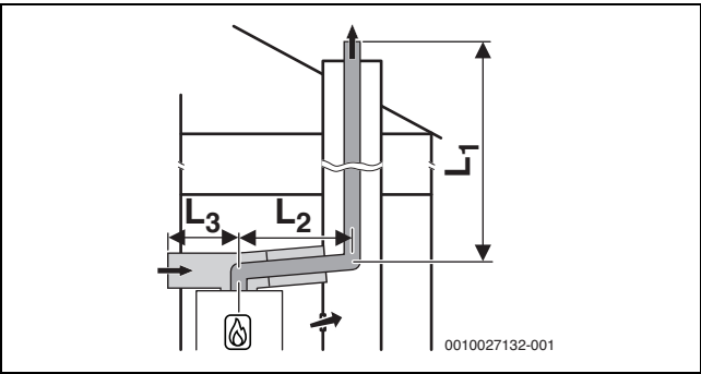
Рис. 22 Схема жесткого отвода дымовых газов согласно C 53x в шахте и схема подачи воздуха/отвода дымовых газов с отдельной линией подвода воздуха и концентрической линией отвода дымовых газов в помещении для установки
