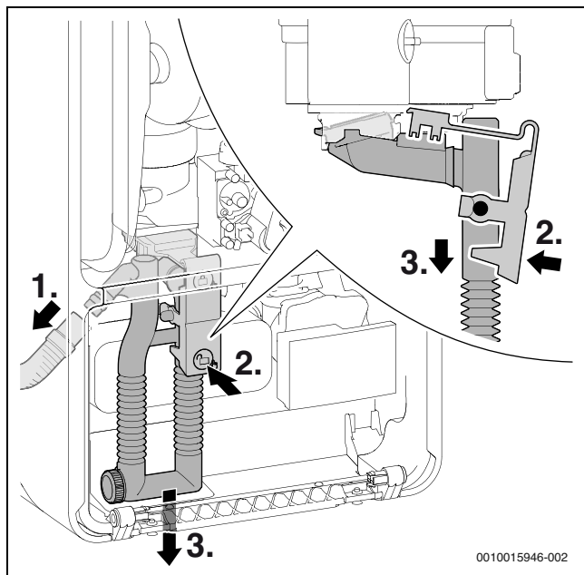
Рис. 90 Демонтаж конденсатного сифона
