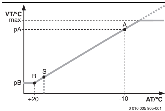
Рис. 112 Отопительная кривая
