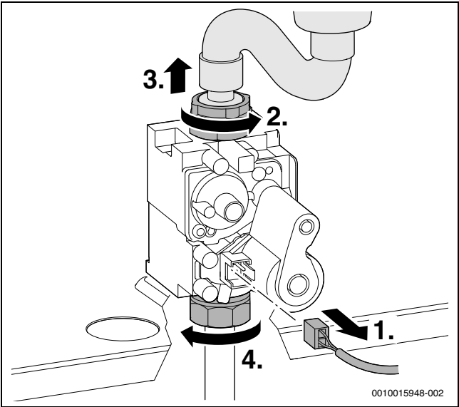
Рис. 99 Извлечение штекера и отвинчивание накидных гаек
