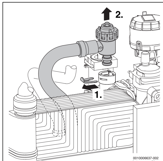
Рис. 96 Демонтаж предохранительного клапана (отопительного контура)
