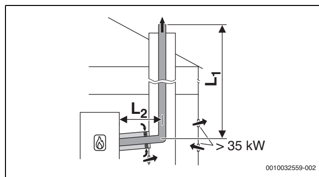
Рис. 49 Схема жесткого отвода дымовых газов в шахте согласно B 33 с забором воздуха из помещения через концентрический подвод воздуха/отвод дымовых газов в помещении для установки
