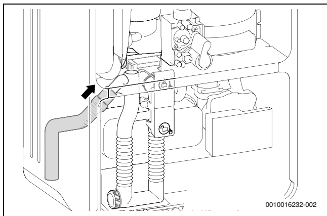
Рис. 64 Подсоединение шланга к сифону для отвода конденсата
