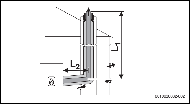
Рис. 17 Концентрическая схема подачи воздуха/отвода дымовых газов согласно C 33x в шахте
