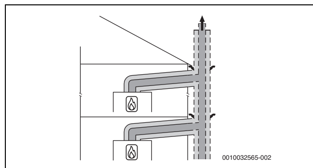
Рис. 53 Подключение нескольких котлов к одному дымоходу согласно C_{(12)3x} с концентрическим подводом воздуха/отводом дымовых газов вне помещения для установки
