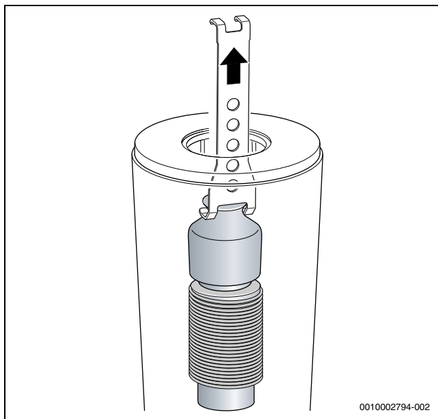
Рис. 85 Выньте верхний рассекатель
