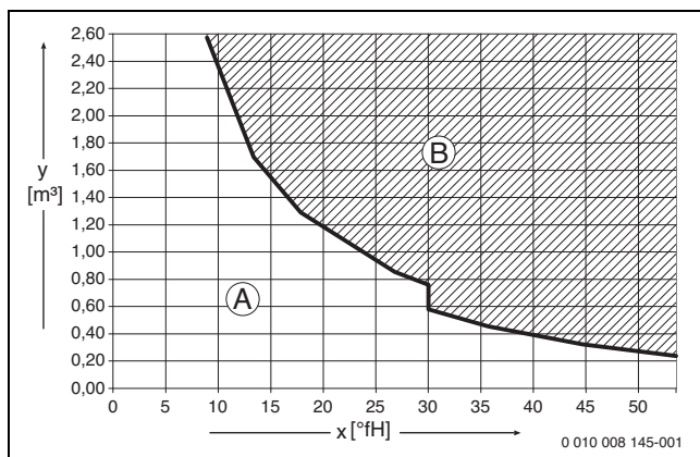
Рис. 60 Требования к воде для заполнения и подпитки в °fH для котлов < 50 кВт
