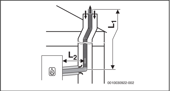
Рис. 33 Схема гибкого отвода дымовых газов согласно C 93x в шахте и концентрический подвод воздуха/отвод дымовых газов в помещении для установки
