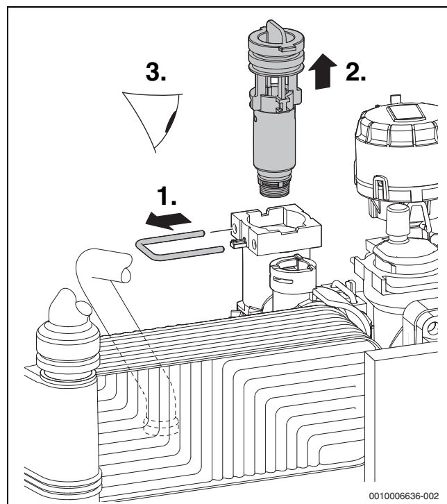
Рис. 97 Проверка сетчатого фильтра в трубе холодной воды
