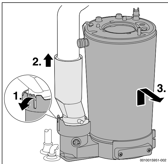
Рис. 105 Демонтаж теплообменника
