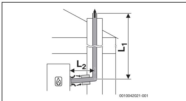
Рис. 45 Жёсткий отвод дымовых газов в шахте по B 53p с забором воздуха из помещения и с концентрическим соединительным элементом между помещением установки котла и шахтой
