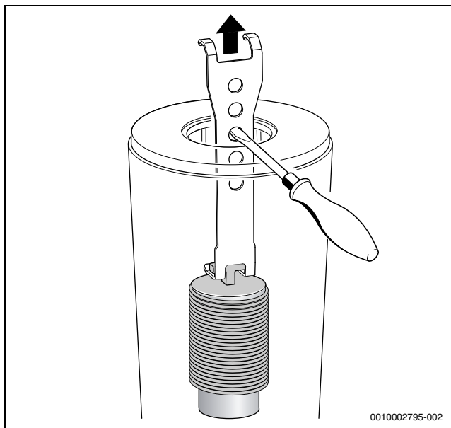
Рис. 86 Выньте нижний рассекатель
