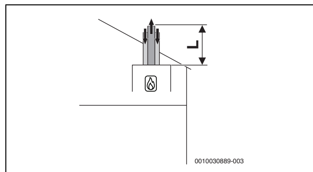
Рис. 14 Вертикальная концентрическая схема подачи воздуха/отвода дымовых газов согласно C 33x
