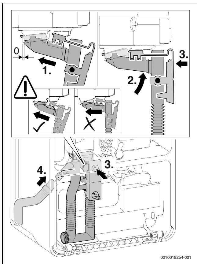
Рис. 95 Установка сифона для отвода конденсата
