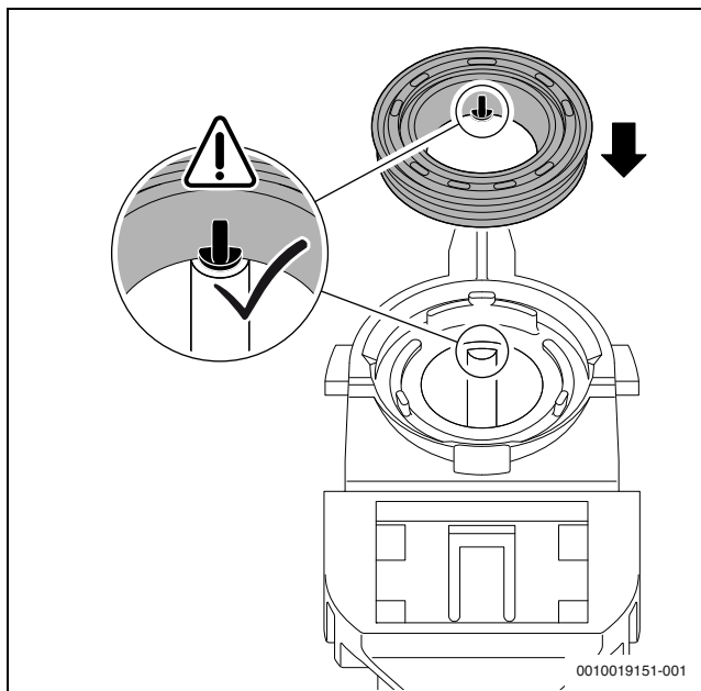
Рис. 93 Выравнивание нового уплотнения на сифоне для отвода конденсата
