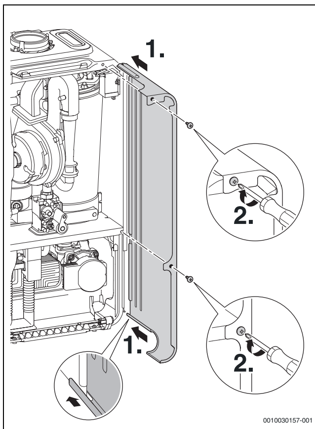
Рис. 108 Установка боковой облицовки
