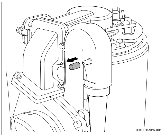
Рис. 80 Измерительный штуцер на смесительном устройстве
