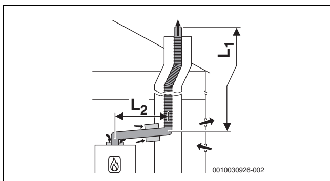
Рис. 46 Схема гибкого отвода дымовых газов в шахте согласно B 53p с забором воздуха из помещения топочной для подвода воздуха и с концентрическим соединительным элементом между помещением для установки и шахтой
