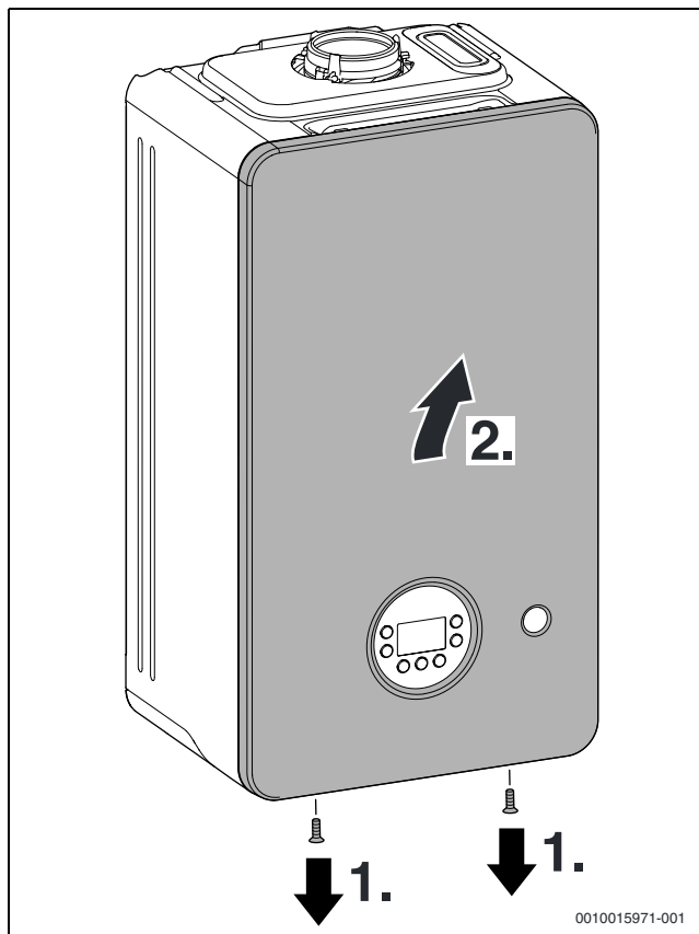
Рис. 62 Снятие передней облицовки
