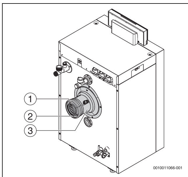
Рис. 38 Установите подсоединение к дымовой трубе
