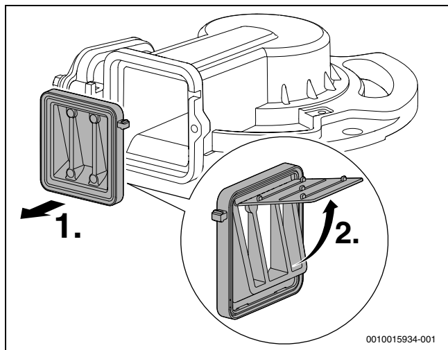
Рис. 83 Обратный клапан в смесительном устройстве
