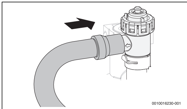
Рис. 63 Подсоединение шланга к предохранительному клапану
