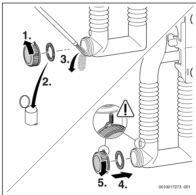
Рис. 91 Чистка конденсатного сифона
