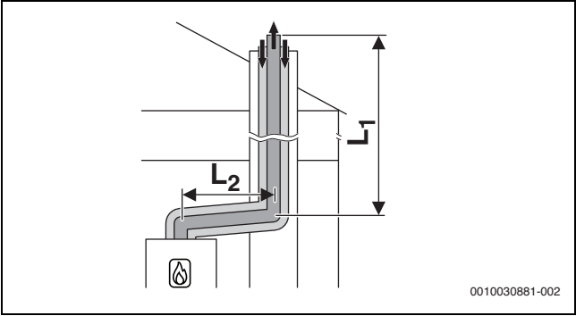
Рис. 16 Концентрическая схема подачи воздуха/отвода дымовых газов согласно C 33x в шахте
