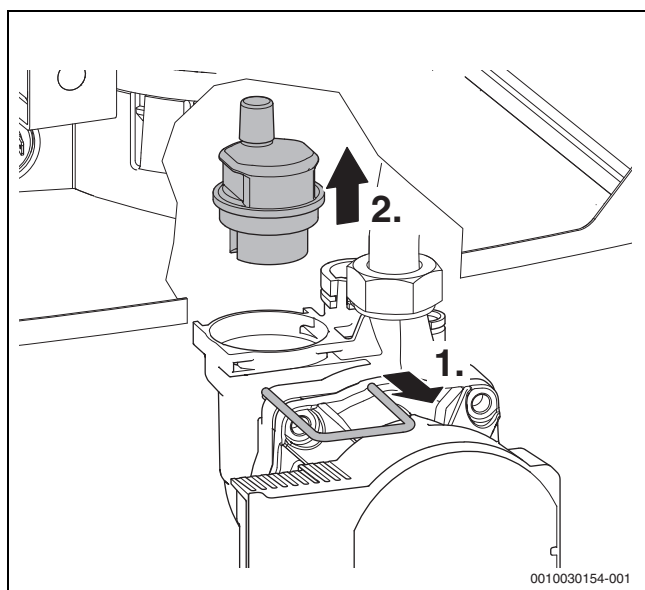
Рис. 102 Демонтаж автоматического воздухоотводчика
