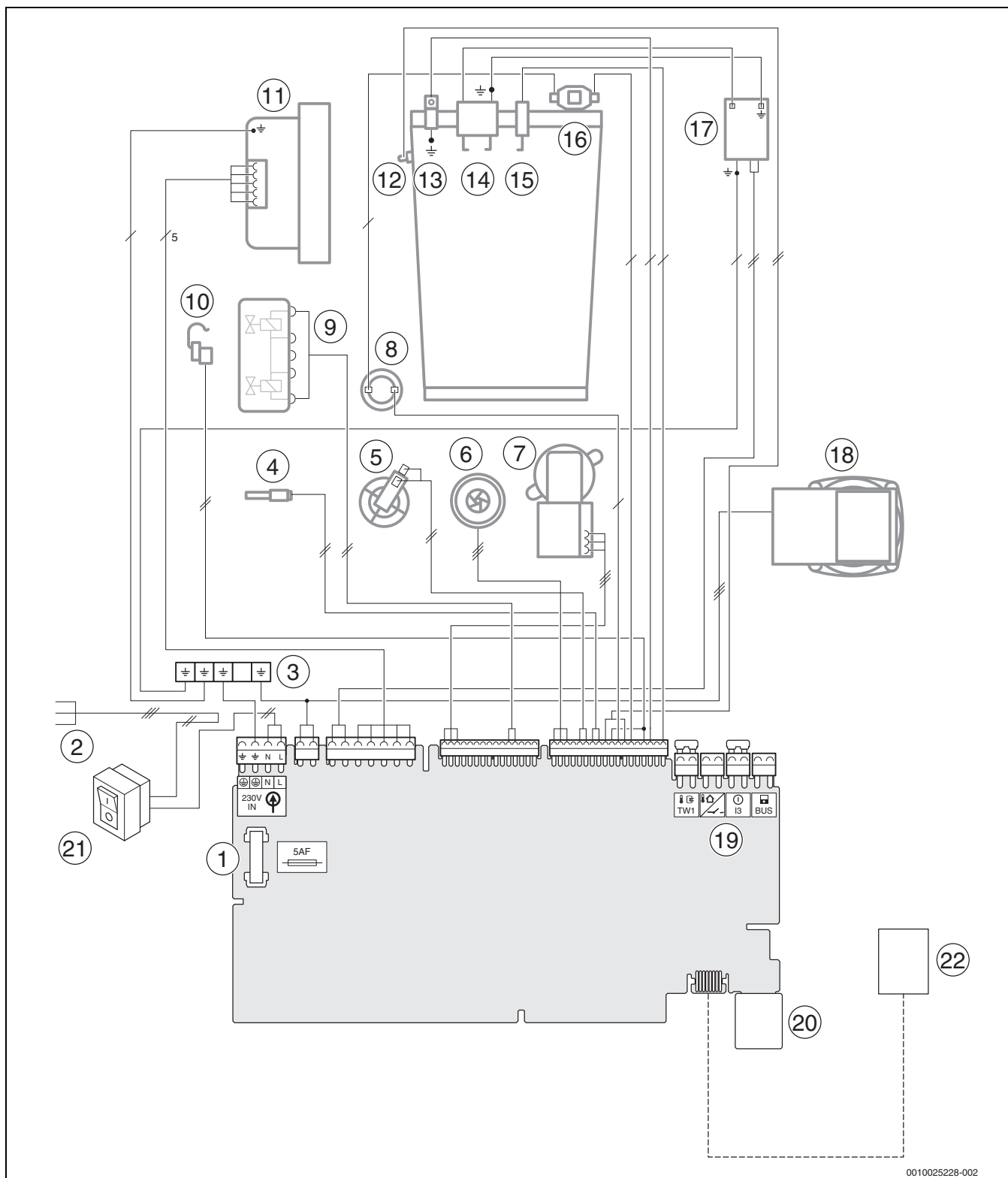
Рис. 111 Электрические соединения
