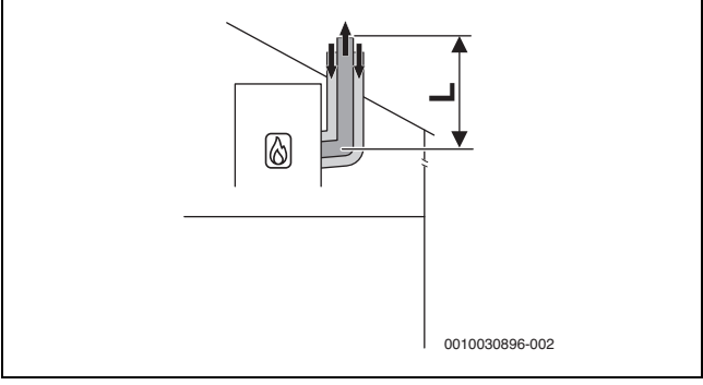
Рис. 19 Вертикальная концентрическая схема подачи воздуха/отвода дымовых газов согласно C 33x
