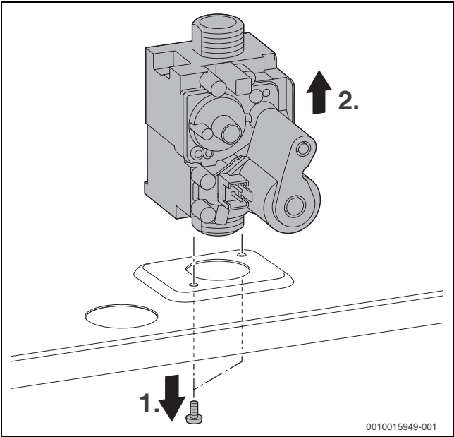
Рис. 100 Демонтаж газовой арматуры
