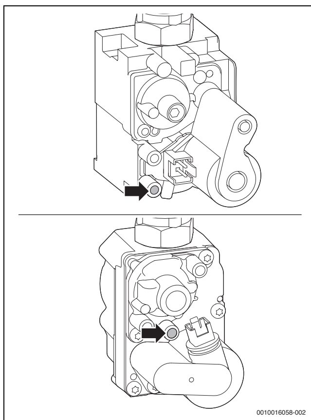
Рис. 78 Штуцер для выполнения замеров давления газа
