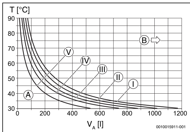
Рис. 61 Характеристики расширительного бака
