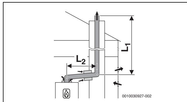
Рис. 39 Жёсткий отвод дымовых газов в шахте по B 53p с забором воздуха из помещения и с концентрическим соединительным элементом между помещением установки котла и шахтой
