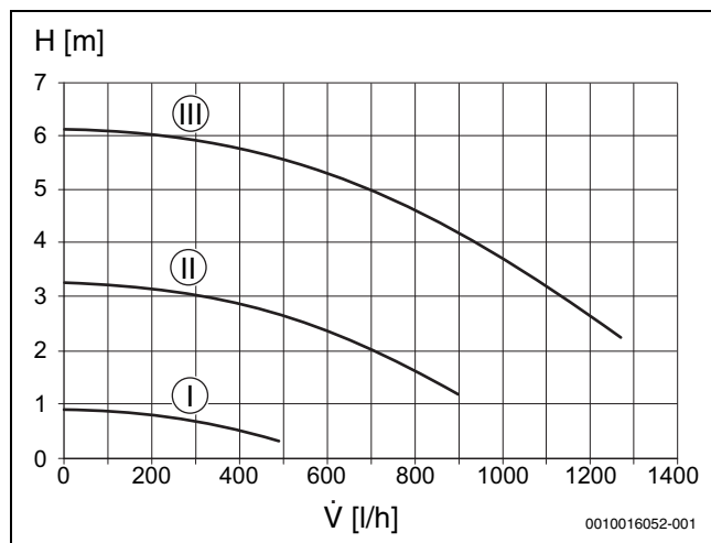
Рис. 73 Характеристическая кривая насоса отопительного контура (постоянная частота вращения)
