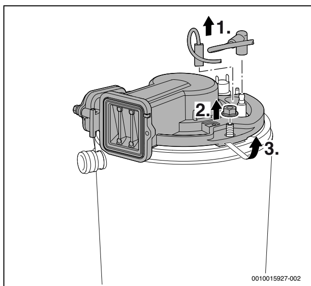
Рис. 82 Снятие крышки горелки
