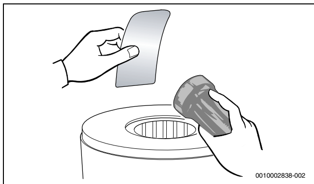
Рис. 88 Проверка наличия грязи в теплообменнике
