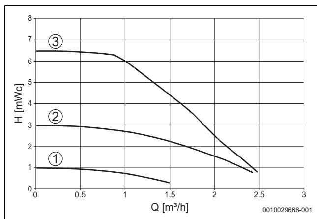
Рис. 74 Характеристическая кривая насоса отопительного контура (постоянное давление)
