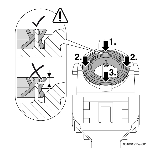
Рис. 94 Прижатие уплотнения
