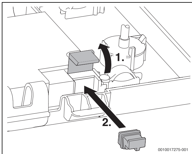
Рис. 107 Вставка кодирующего штекера
