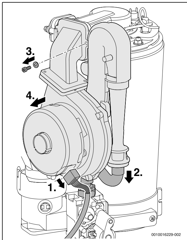
Рис. 81 Демонтаж вентилятора со смесительным устройством
