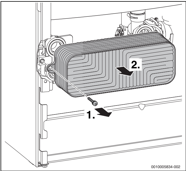
Рис. 98 Демонтаж пластинчатого теплообменника
