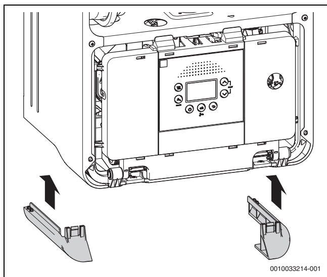
Рис. 109 Установка боковых пластиковых планок
