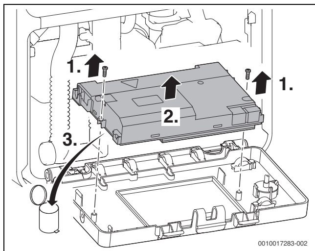
Рис. 106 Замена электронного блока котла
