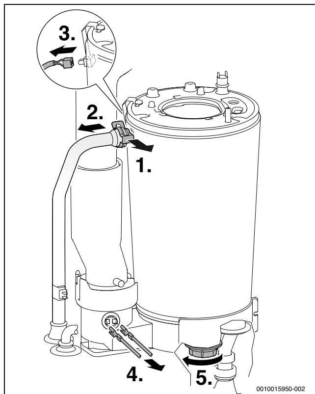
Рис. 104 Отсоедините трубу подающей линии и провода
