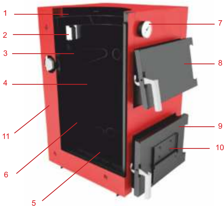
Малюнок 2 - Зовнішній вигляд та основні елементи котла
