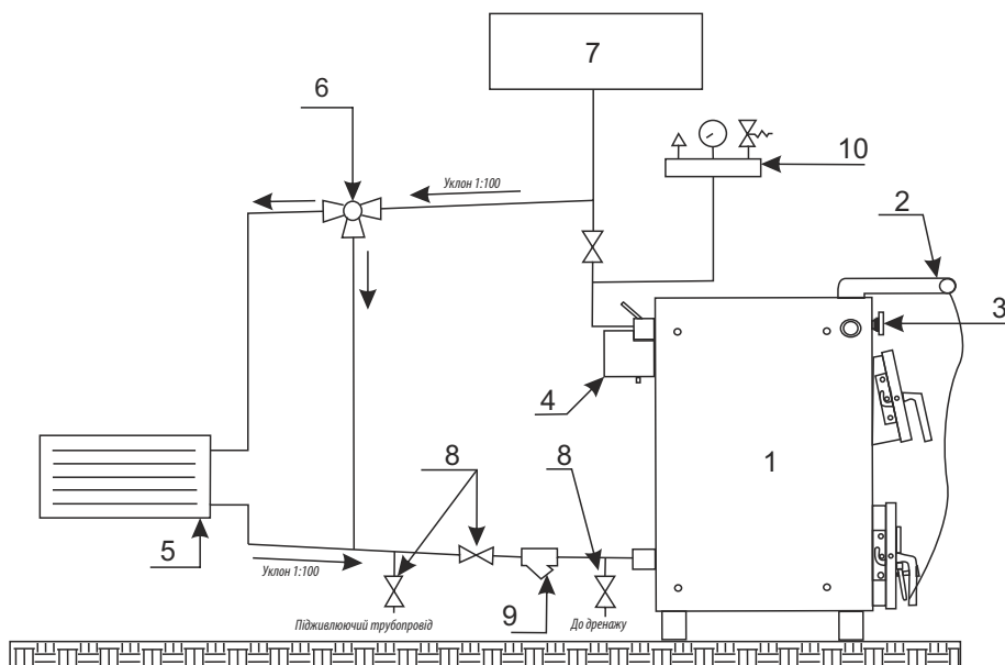
Малюнок 4 – Схема підключення котла до системи опалення з природною циркуляцією теплоносія
