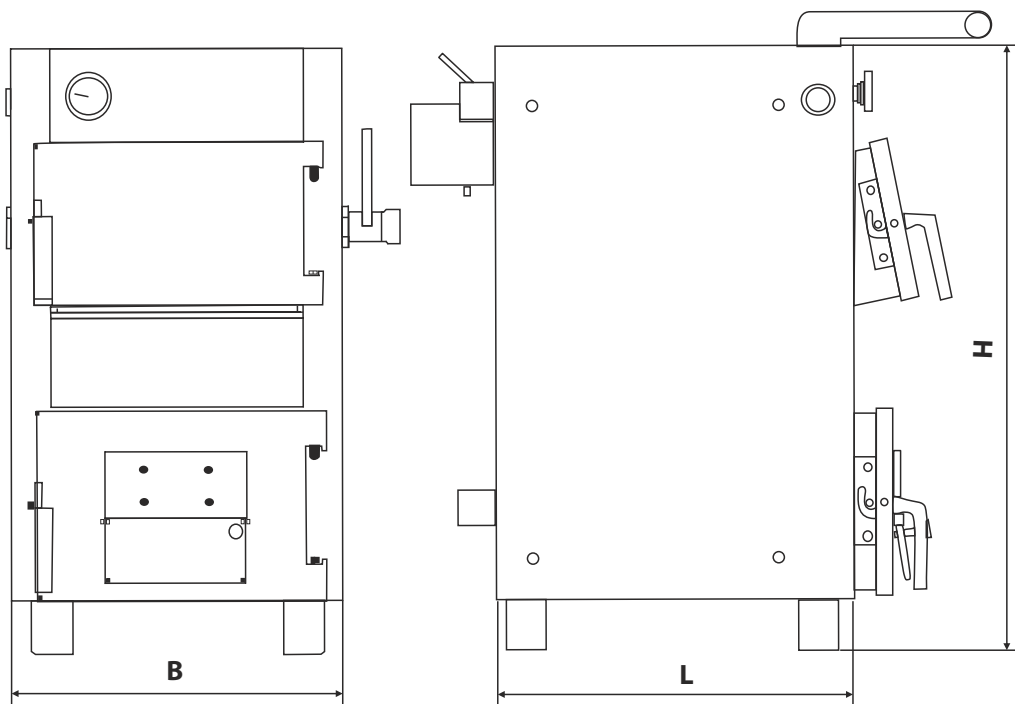
Малюнок 1 – Габаритне креслення котла типу Marten Base.
