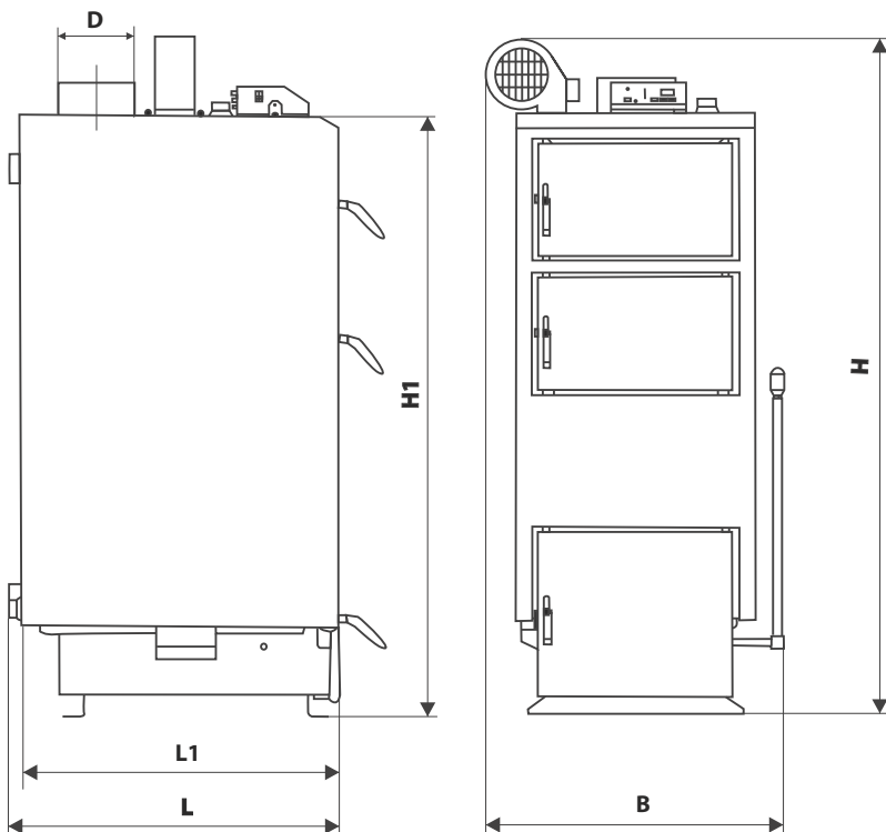
Малюнок 1 – Габаритне креслення котла типу Marten Comfort
