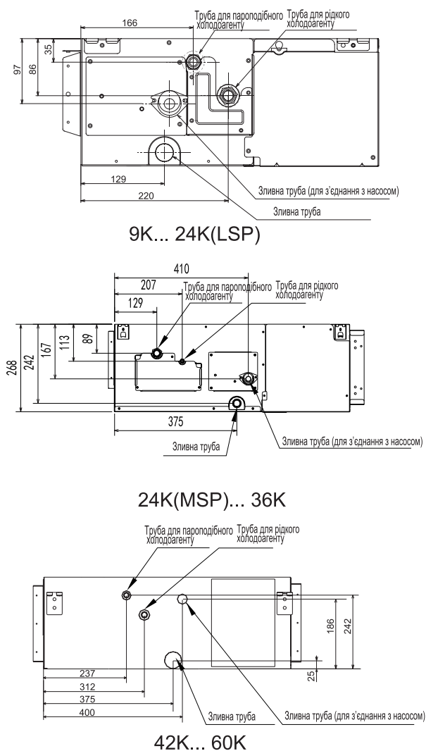
Рис. 4.1. Точки з'єднання труб (одиниця вимірювання: мм)
