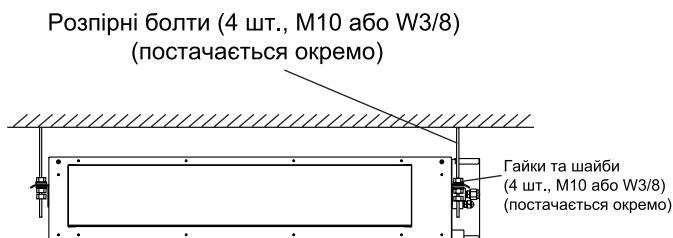
Рис. 3.4. Встановлення внутрішнього блоку
