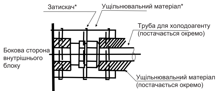
Рис. 4.4. Процедура ізолювання труб
