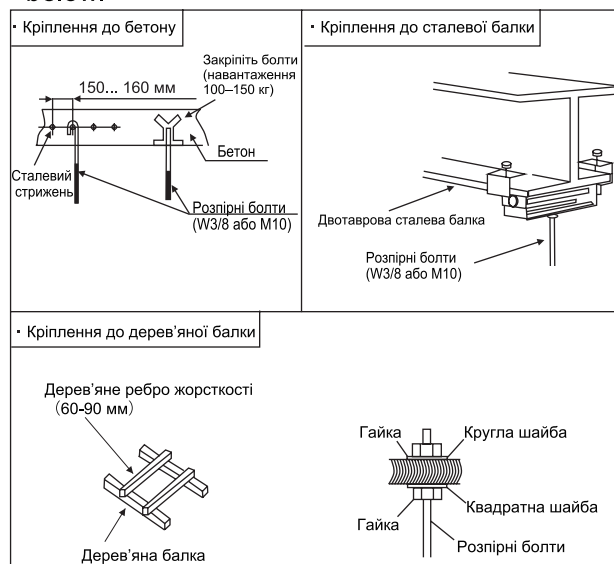
Рис. 3.2.1 Кріплення розпирних болтів
