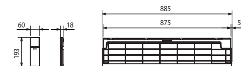
ИК-пульт управления SG15D
