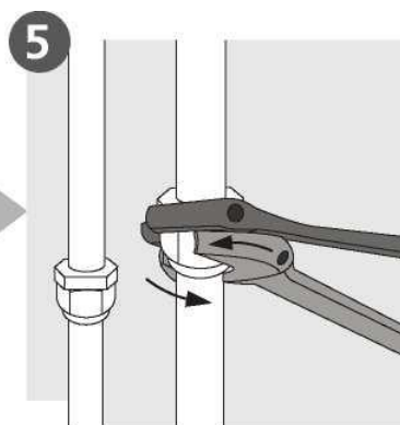
З'єднання трубопроводу
