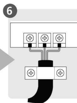
Під'єднання кабелю
