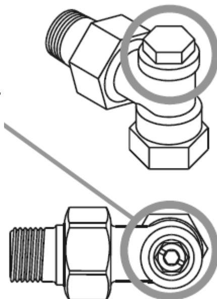
Рис. 5. Идентификация Verafix.
