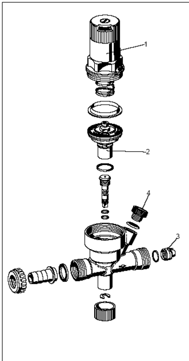
Запасные части к питающему клапану VF06 (выпуска 1998 года или позже)
