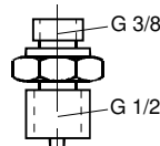
Стальной фитинг для манометра G \frac{3}{8} - G \frac{1}{2} Тип: H 124-114 № 0403 358 Вес: ~0.18 кг
