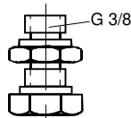
Стальной фитинг Ermeto для стальной трубы Ø 10 мм Тип: R-AD 10-FN 43 № 0405 478 Вес: ~0.1 кг
