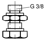
Стальной фитинг Ermeto для стальной трубы Ø 6 мм Тип: R-AD 6-FN 43 № 0405 466 Вес: ~0.1 кг
