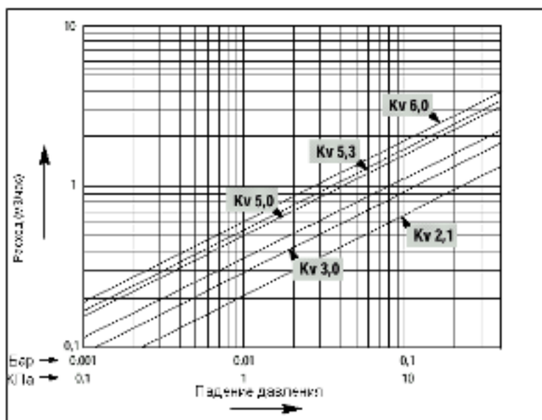
Рис 8. Характеристика падения давления на 2-х ходовом клапане
